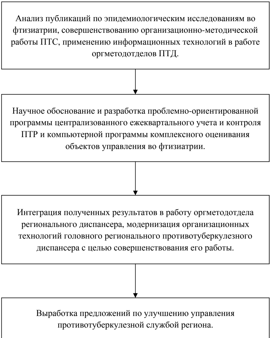
Рис. 1. Алгоритм исследования
